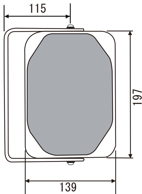
《取り付け穴位置》
