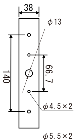
《取り付け穴位置》
